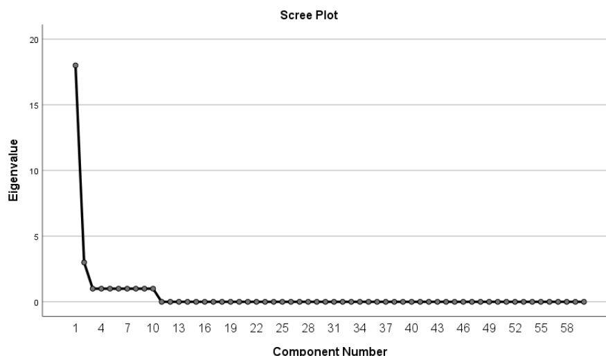
نمودار ۲-۴ نمودار سنگ‌ریزه‌ای برای تخمین تعداد عامل‌ها
