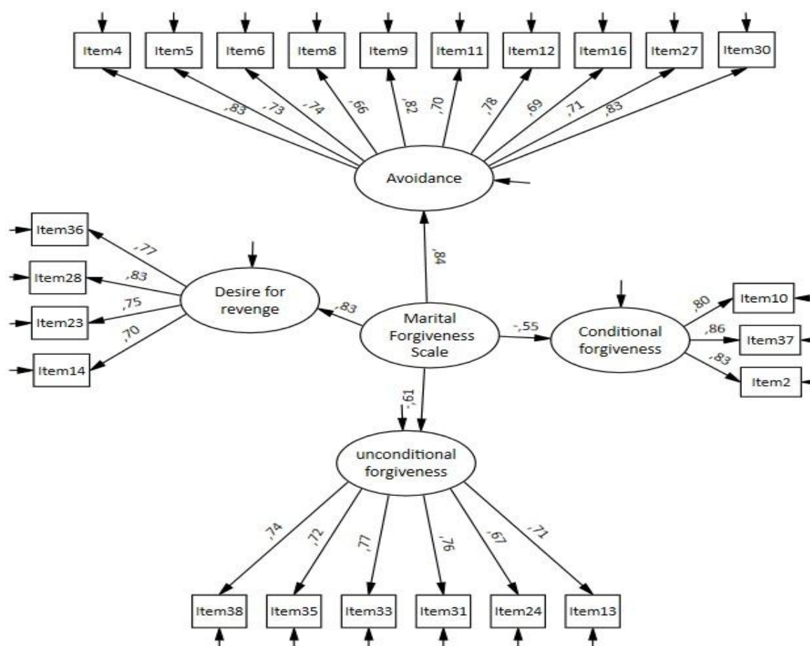
شکل ۲ مدل CFA مرتبه دوم
